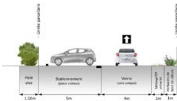
Figure 41 : vues en coupe des profils de voirie (n°1, 2 et 4)
