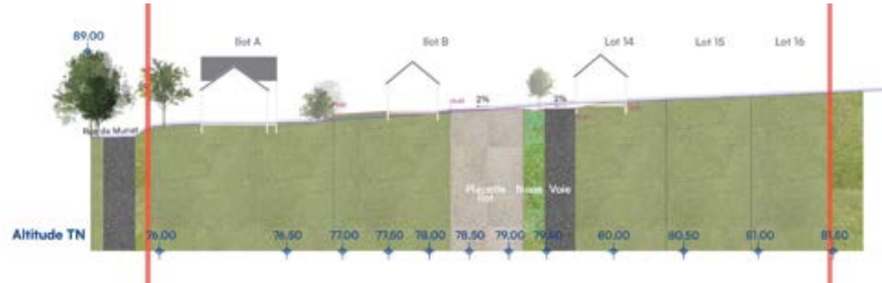
Figure 46 : vue en coupe du quartier du Racoupeau BB'
